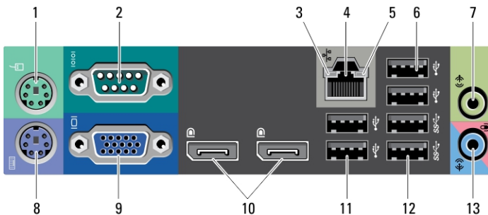
Abbildung 5. Rückansicht des Kompaktgehäuses
