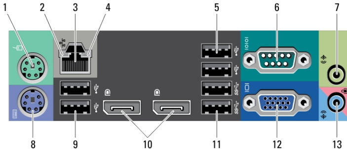
Abbildung 3. Rückansicht von Mini-Tower und Desktop-PC
