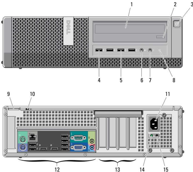
Abbildung 2. Vorder- und Rückansicht des Desktop-PCs
